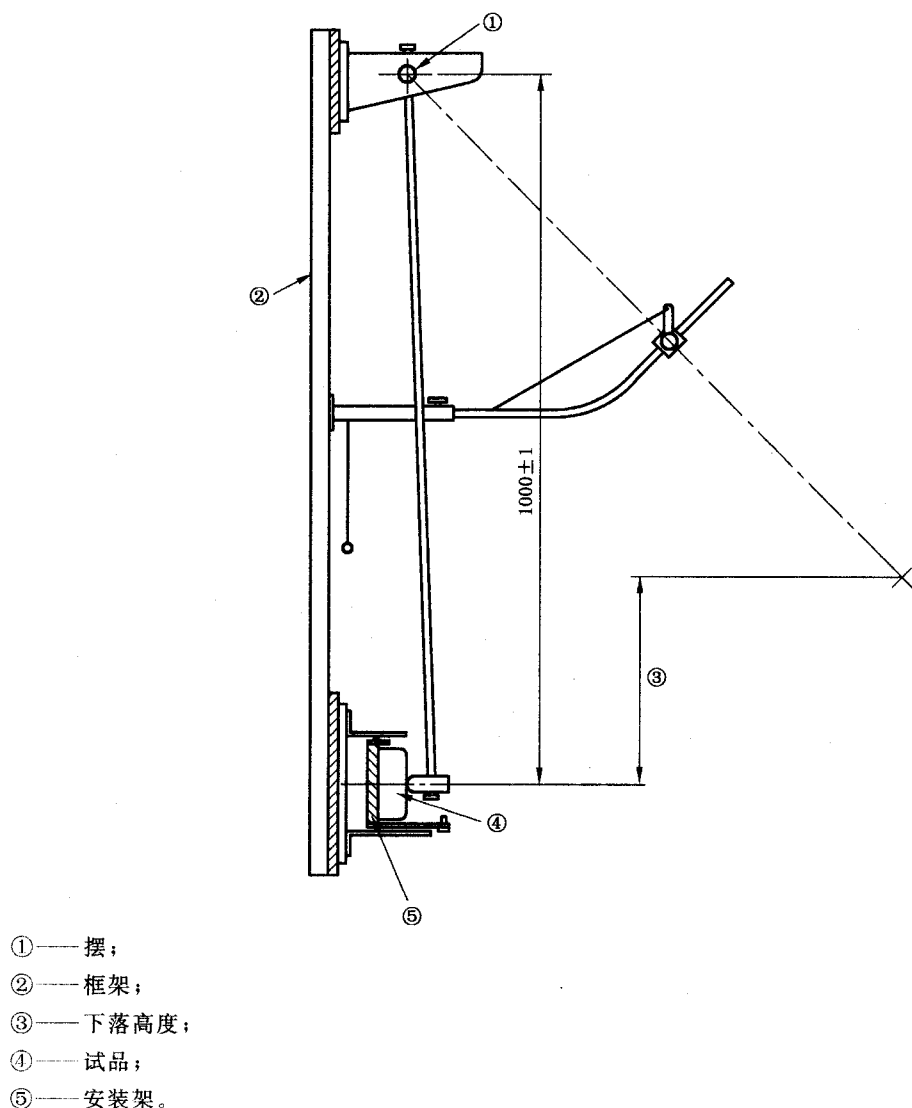
a) 试验装置
